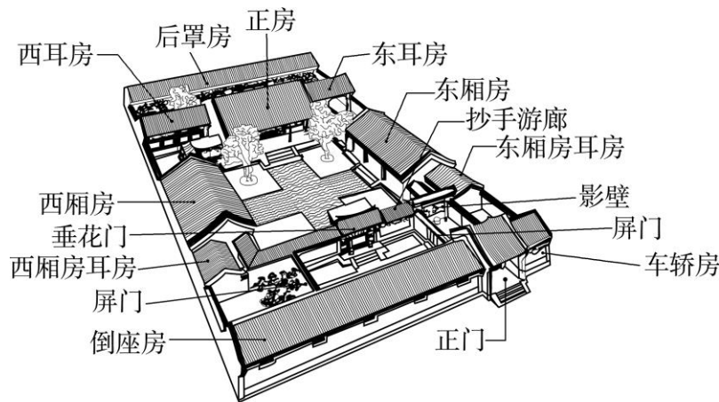
三进四合院鸟瞰图
